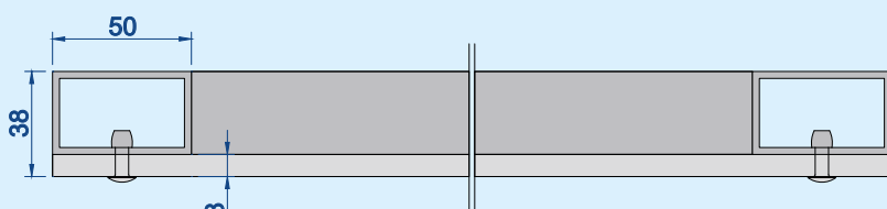
Horizontalschnitt: Maßstab 1:3
