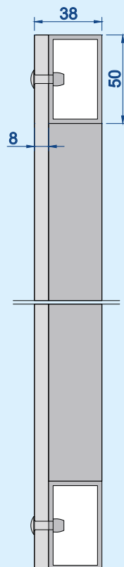
Vertikalschnitt: Maßstab 1:3
