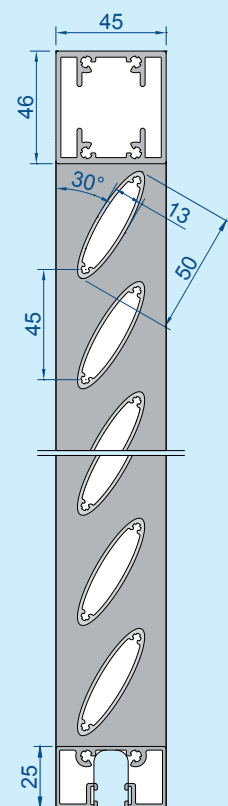
Vertikalschnitt: Maßstab 1:3
