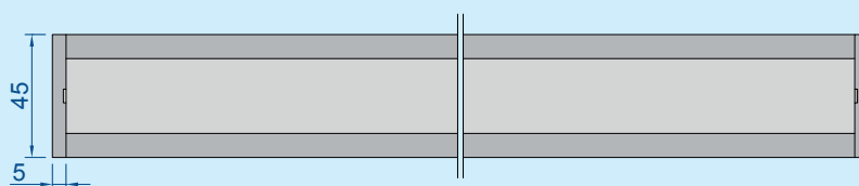
Horizontalschnitt: Maßstab 1:3
