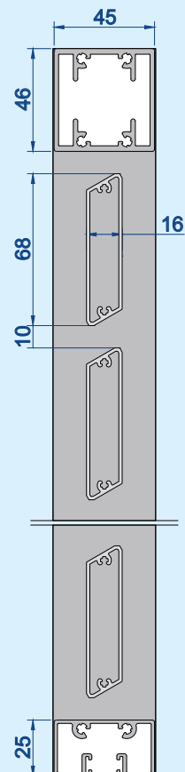
Vertikalschnitt: Maßstab 1:3
